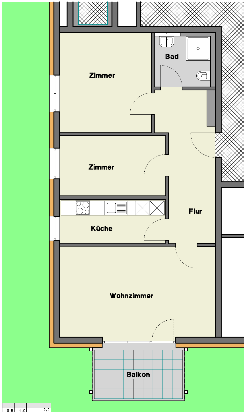
Wohnungen 4 / 8 / 12 und 16 Typ rechts vorne, 3 Zimmer, Wohnfläche ca. 77 qm
